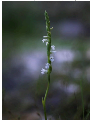
Fig. 20. Spiranthes aestivalis (Moralzarzal, 25-VI-2022, HMA).
