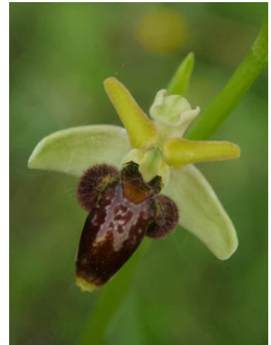
Fig. 21. Ophrys cf. × nouletii (Sierra de Guadarrama, 26-V-2025, R. Martínez Pesquera).
